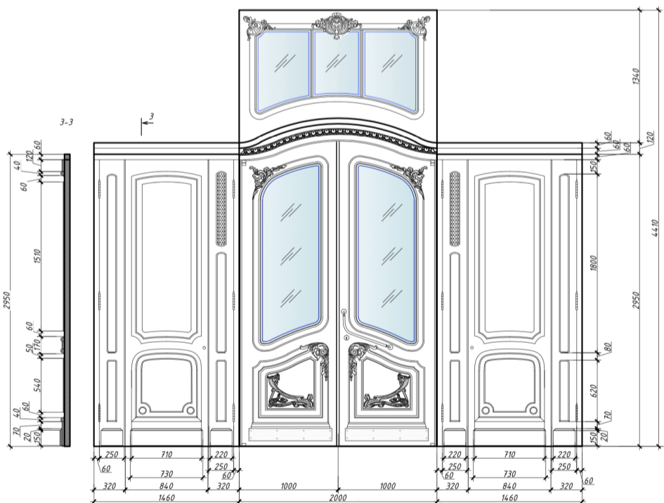
Дом Бака, внутренние двери тамбура парадной №1 – проект
